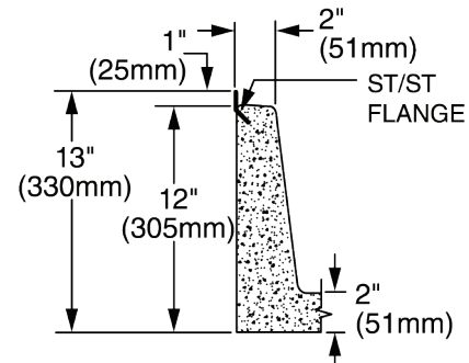
OPTIONAL ST/ST TILING FLANGE
